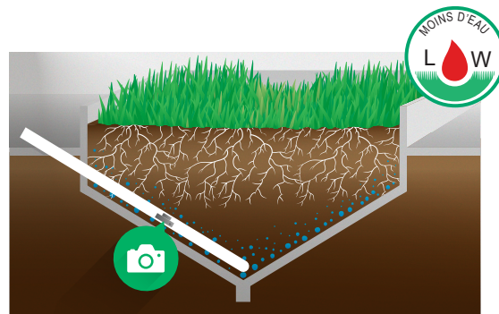
RADIMAX : Système unique au monde d'observation de la densité et de la profondeur des racines.
